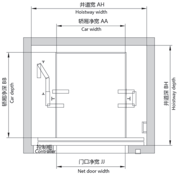
井道布置图 Hoistway plan
