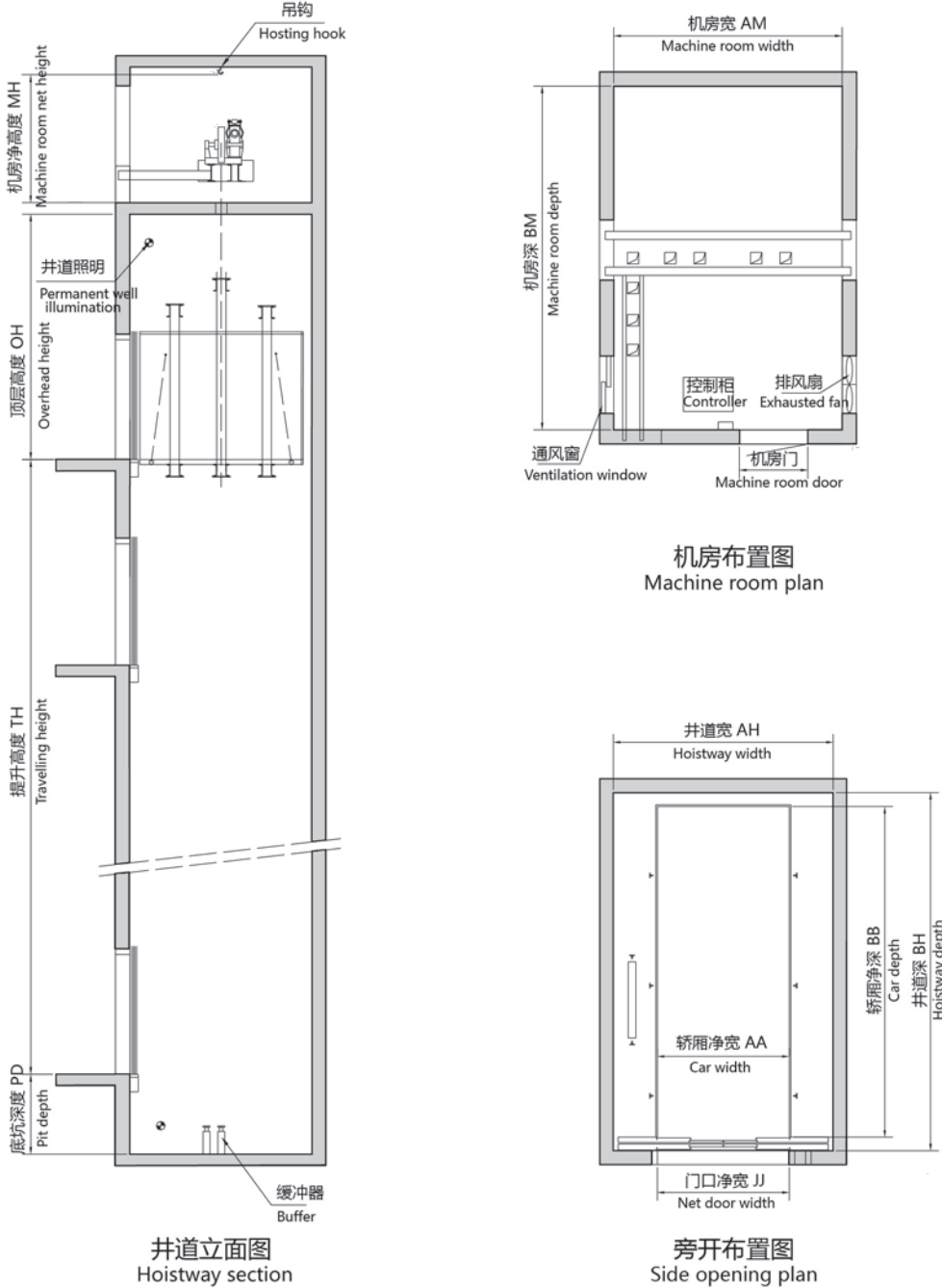
KLQ/VF 汽车电梯参数表 KLQ/VF Car elevator parameter table
