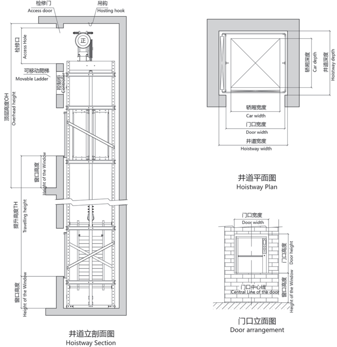
KLZW 杂物电梯参数表 KLZW Dumbwaiter elevator parameter table
